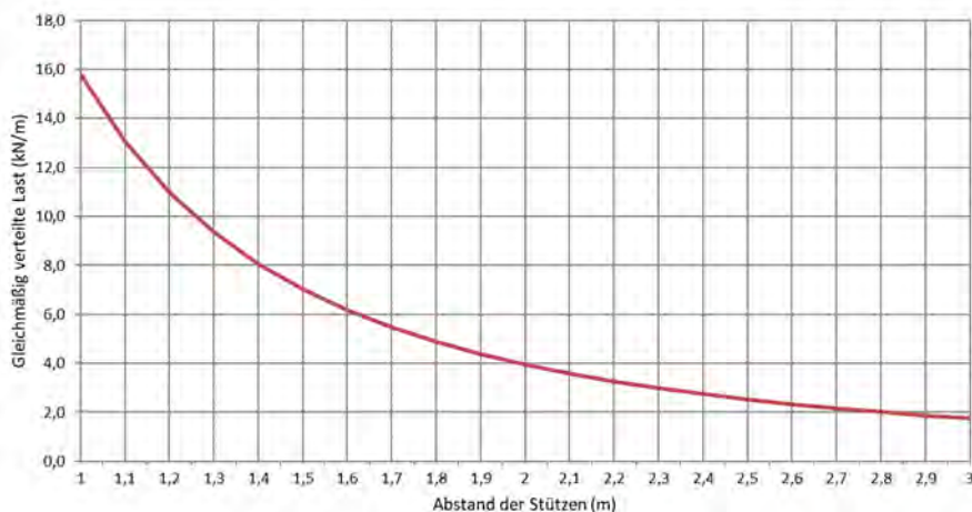
Zulässige Belastung KL 100/400 d=1,5mm (kN/m)
