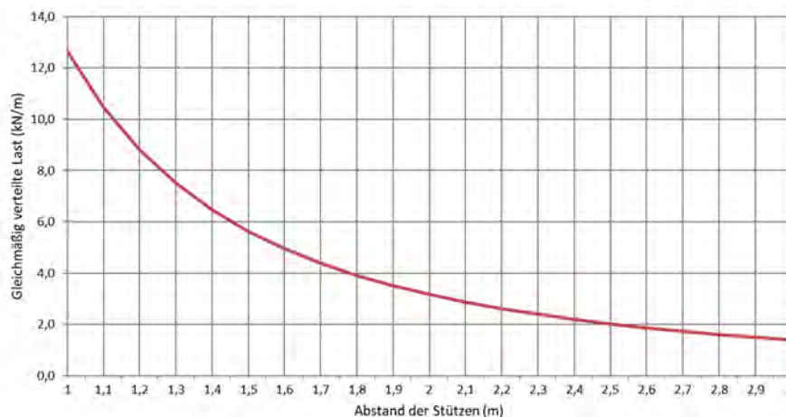
Zulässige Belastung KL 100/300 d=1,5mm (kN/m)
