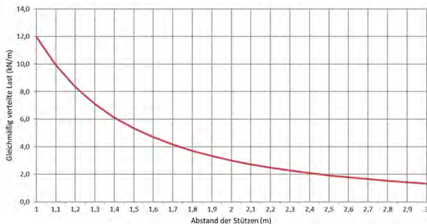
Zulässige Belastung KL 100/200 d=1,5mm (kN/m)
