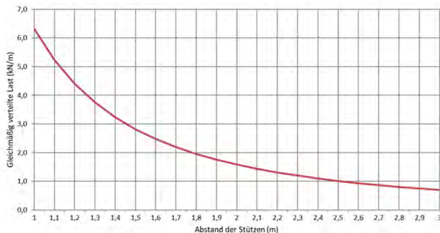
Zulässige Belastung KL 100/100 d=1,0mm (kN/m)
