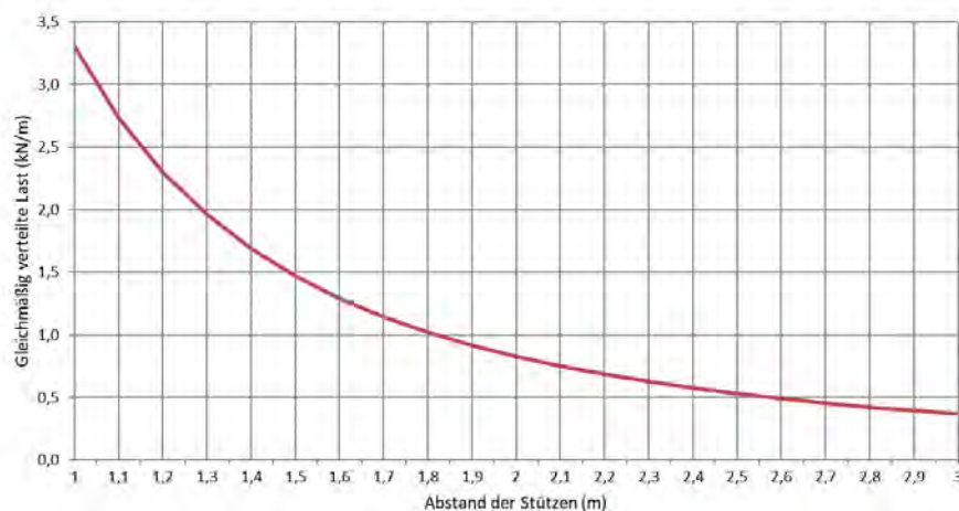
Zulässige Belastung KP 60/500 d=0,8mm (kN/m)
