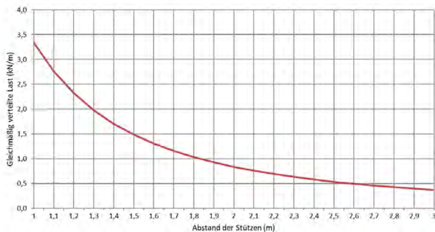
Zulässige Belastung KP 60/400 d=0,8mm (kN/m)
