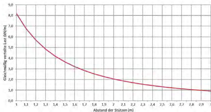
Zulässige Belastung KP 60/300 d=1,5mm (kN/m)
