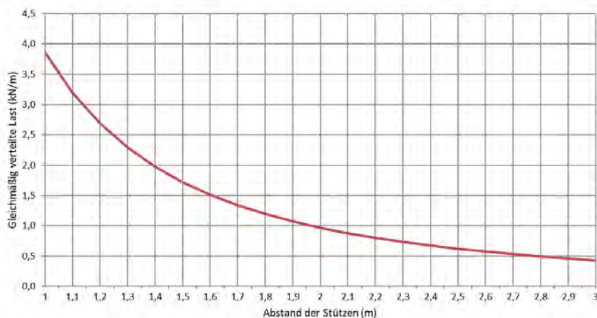
Zulässige Belastung KP 60/600 d=0,9mm (kN/m)
