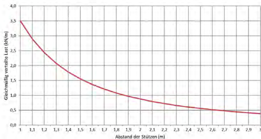
Zulässige Belastung KP 60/500 d=0,9mm (kN/m)
