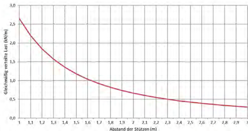
Zulässige Belastung KP 60/300 d=0,75mm (kN/m)
