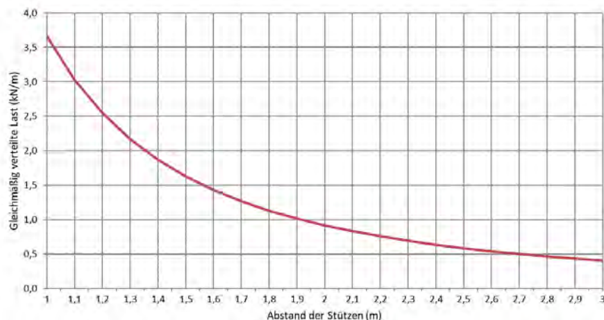
Zulässige Belastung KP 60/200 d=0,75mm (kN/m)
