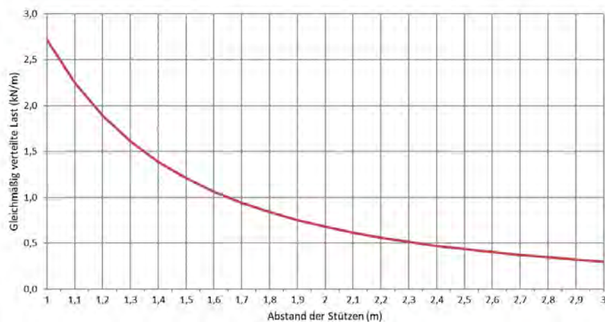
Zulässige Belastung KP 60/100 d=0,75mm (kN/m)
