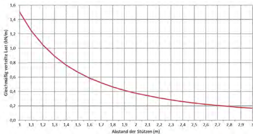
Zulässige Belastung KP 60/200 d=0,6mm (kN/m)
