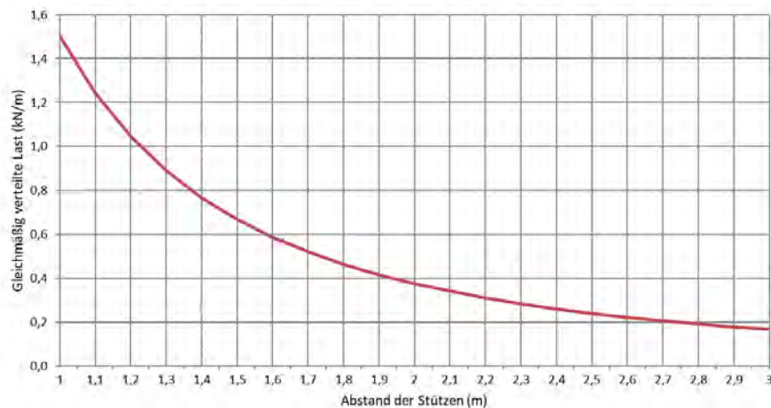
Zulässige Belastung KP 60/100 d=0,6mm (kN/m)
