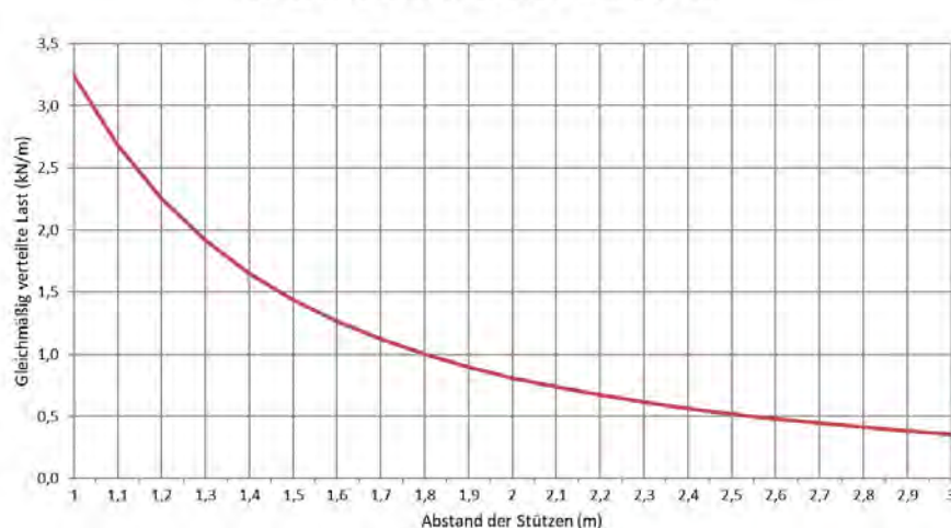
Zulässige Belastung KP 60/600 d=0,8mm (kN/m)
