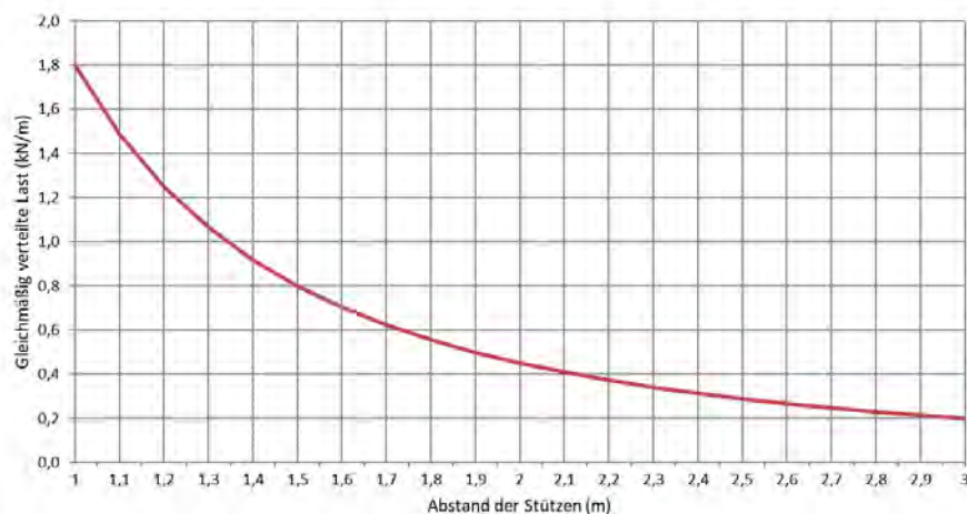
Zulässige Belastung KPA 60/400 d=1,0mm (kN/m)
