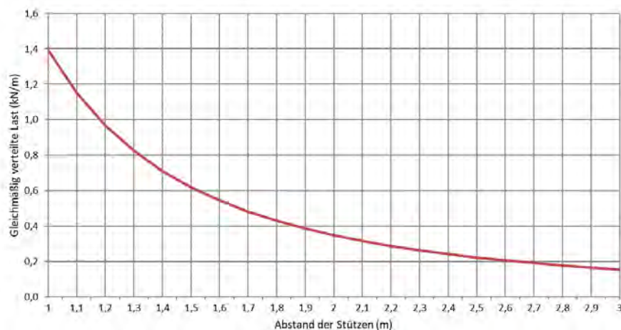
Zulässige Belastung KPA 60/300 d=1,0mm (kN/m)
