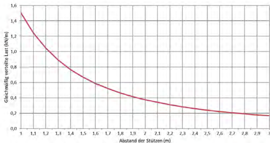
Zulässige Belastung KPA 60/200 d=1,0mm (kN/m)
