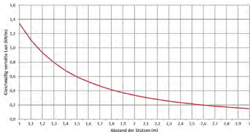
Zulässige Belastung KPA 60/100 d=1,0mm (kN/m)
