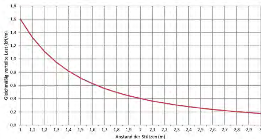
Zulässige Belastung KPA 60/600 d=1,0mm (kN/m)
