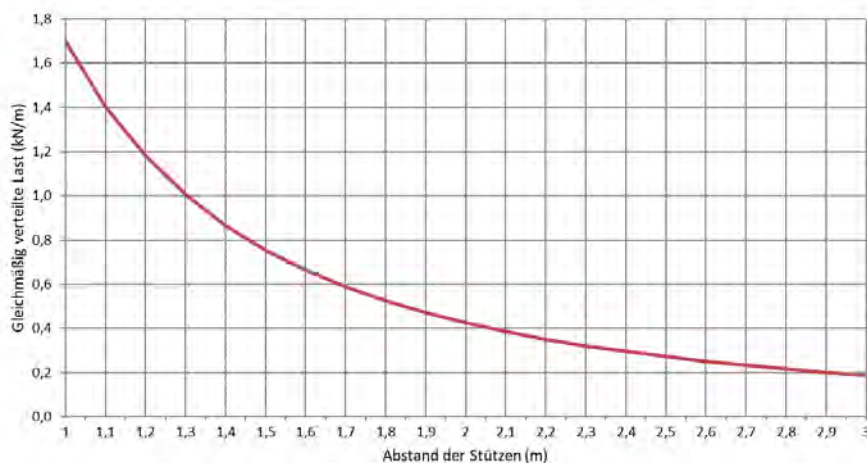
Zulässige Belastung KPA 60/500 d=1,0mm (kN/m)
