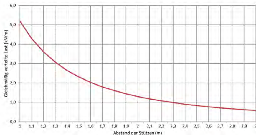
Zulässige Belastung KLA 60/600 d=2,0mm (kN/m)
